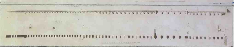
Dibujos del templo de Marte y del puente sobre el Guadiana. De una lámina de Laborde.
